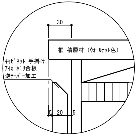
※1 キャビネット 手掛け部分詳細図
