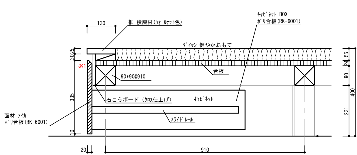
棚下収納 断面詳細図 1/10
