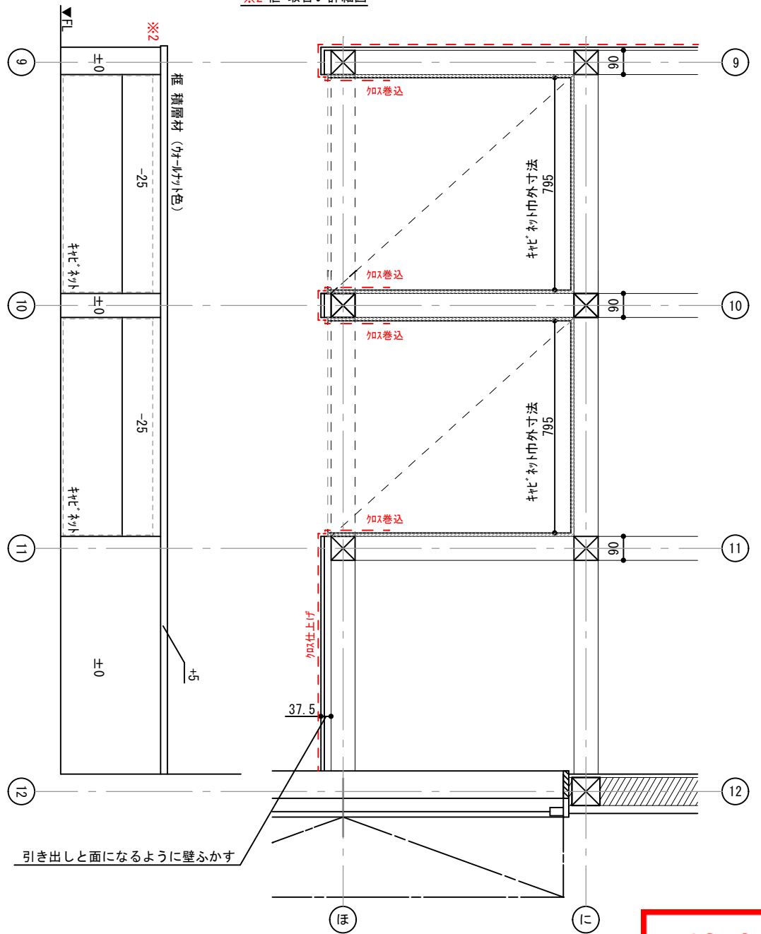
角コーナー 平面詳細図 1/20
