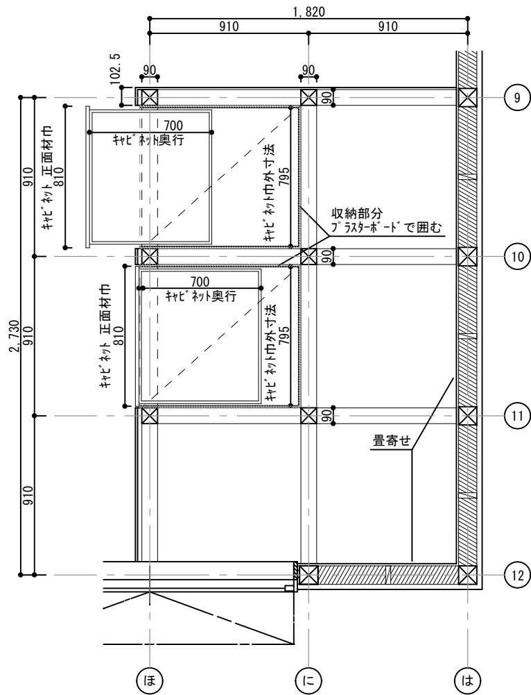
角コーナー 平面詳細図 1/30
